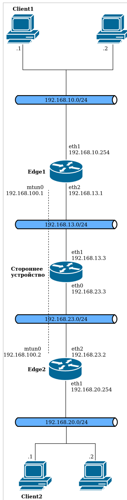
Рисунок 80 – Схема стенда
