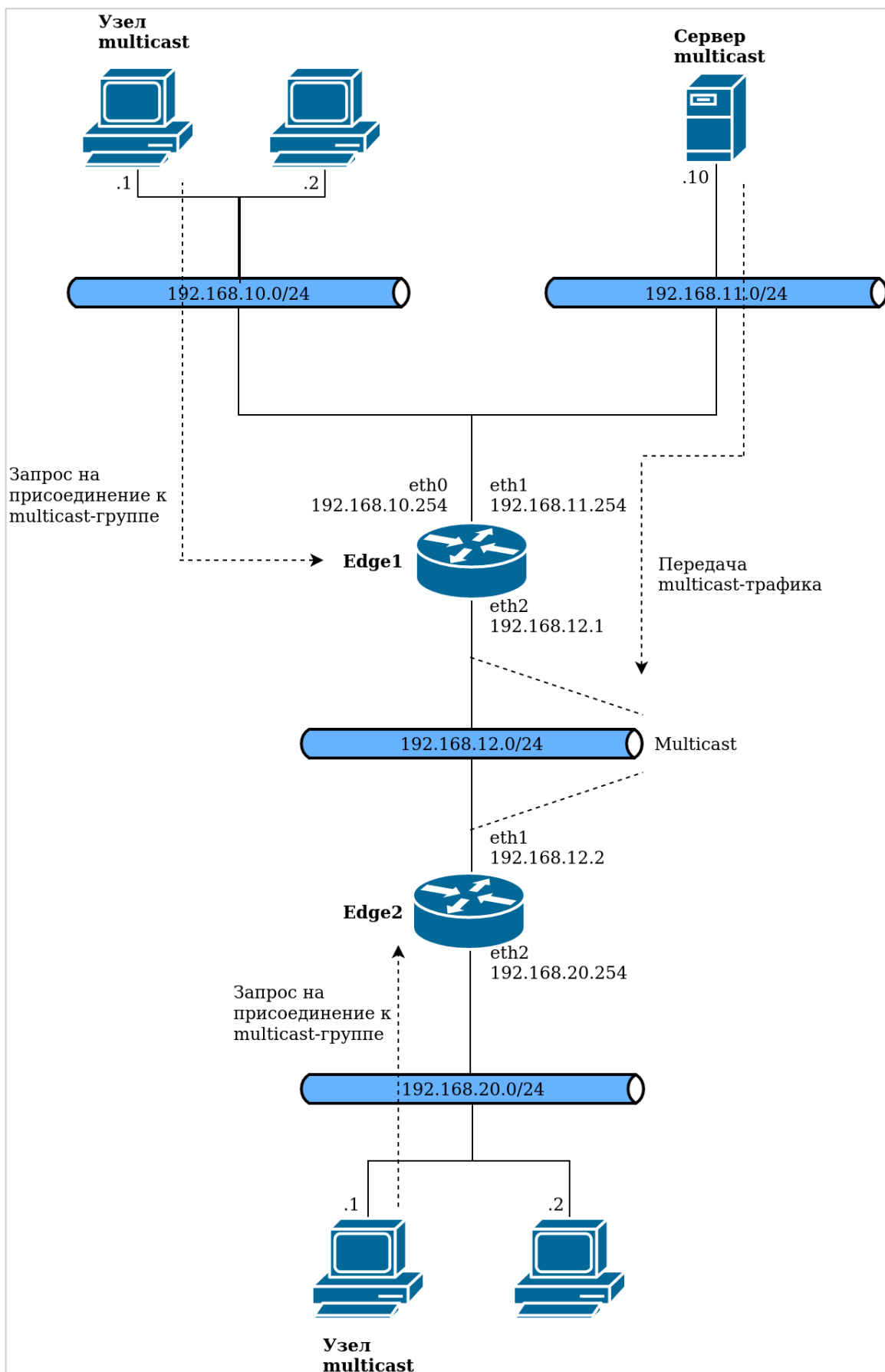
Рисунок 78 – Схема стенда
