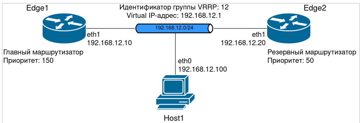
Рисунок 51 – Базовая конфигурация
