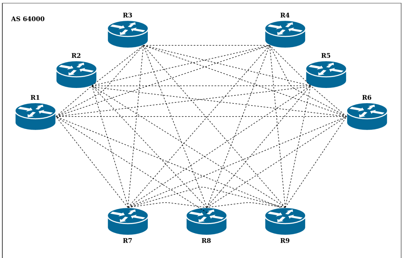
Рисунок 61 – Схема соединения iBGP «каждый с каждым».
