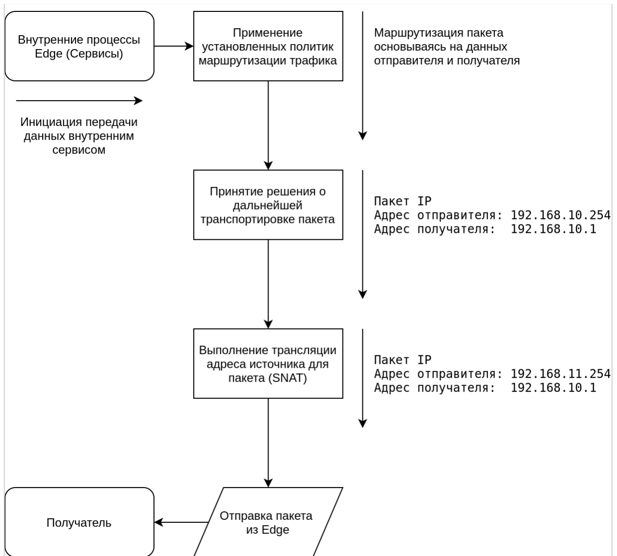
Рисунок 42 – Прохождение трафика, направленного из локальной системы
