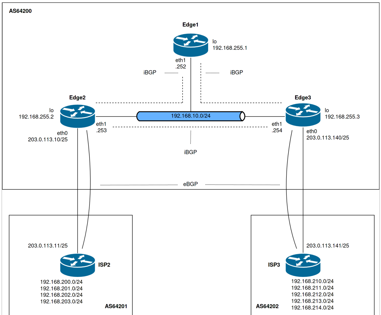
Рисунок 64 – Схема настройки BGP
