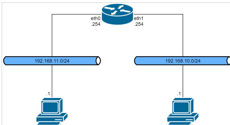
Рисунок 38- Базовая схема
